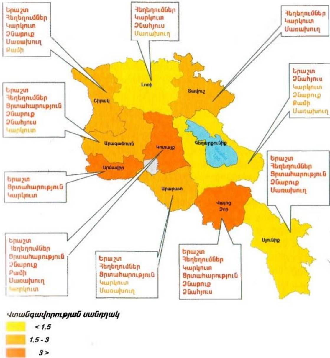
Նկար 5. Հայաստանի մարզերի խոցելիությունը հիդրոօդերևութաբանական վտանգավոր երևույթների նկատմամբ՝
